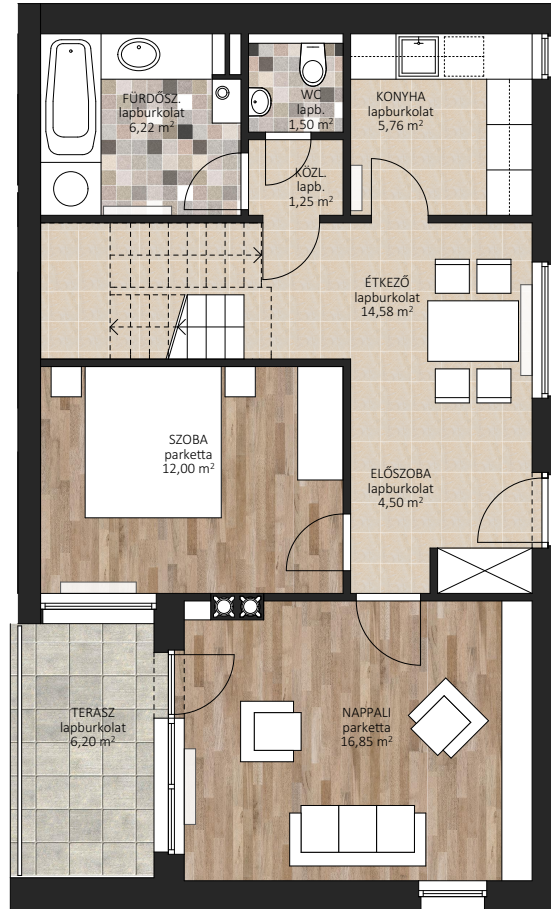
Bejárati szint
